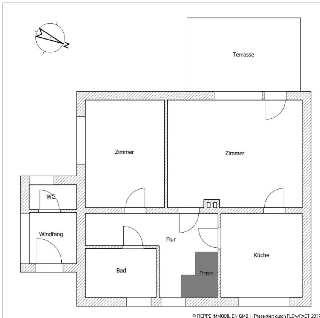
Grundriss Erdgeschoss
