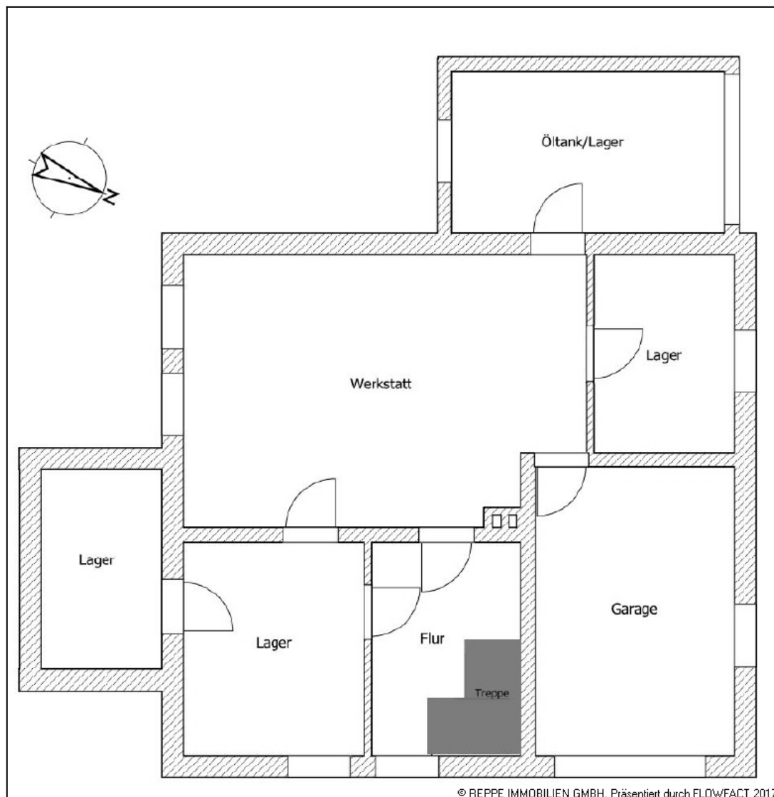
Grundriss Kellergeschoss
